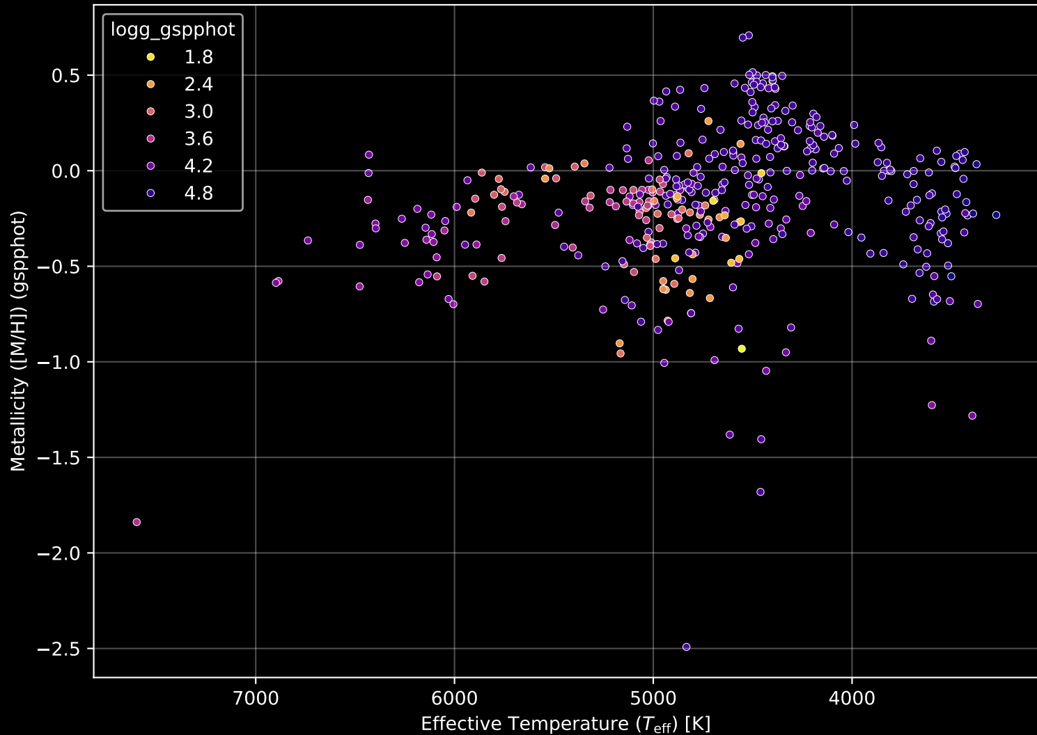
APOGEE DR17 Field: [000+75] Stellar Population Parameters (n= 419)
